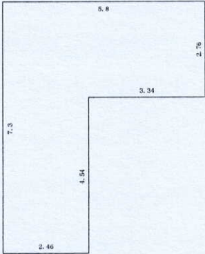
顶层
