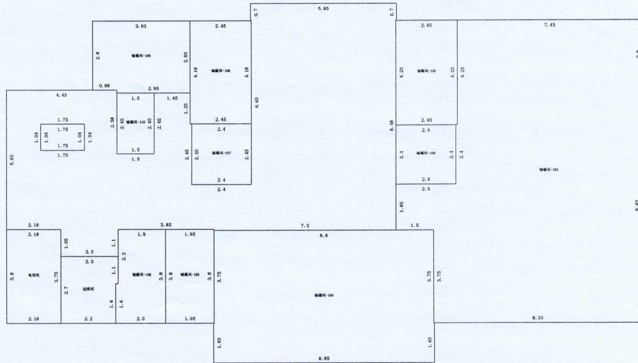
第1层
