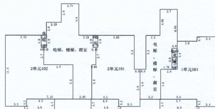
第1层
