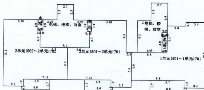
第15~17层
