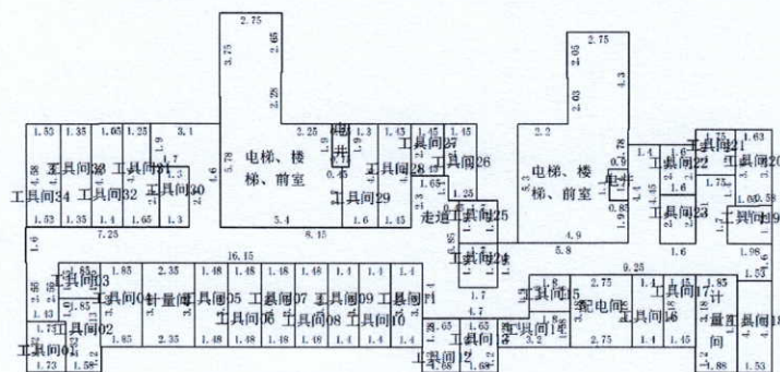
第1层
