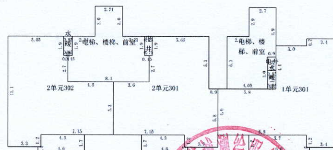
第3层
