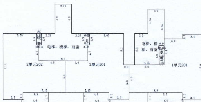
第2层
