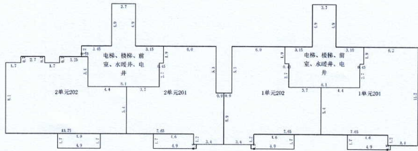
第2层
