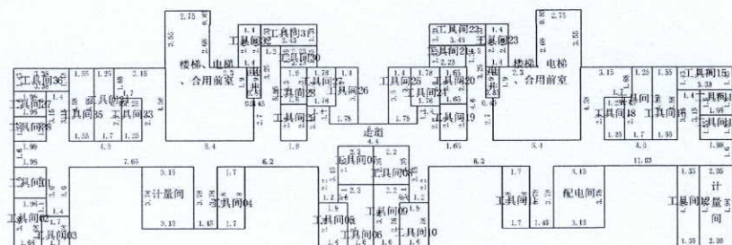
第1层
