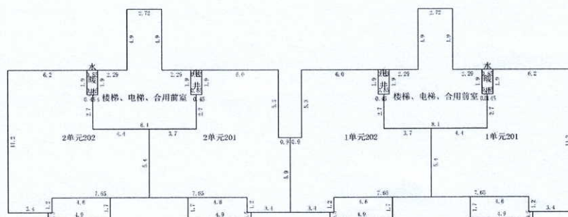
第2层
