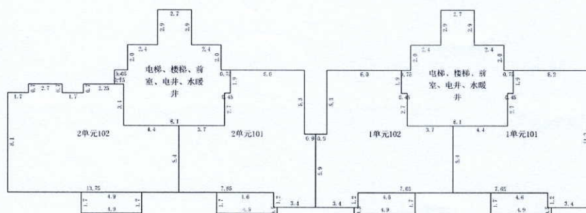
第1层
